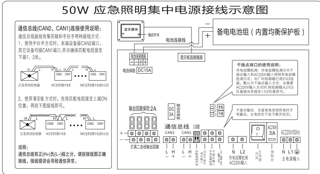
(1)、用户接线示意图 (如图4.1、图4.2)
