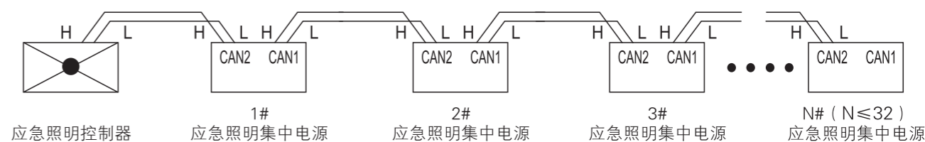
菊花链连接方式示意图（图1）
