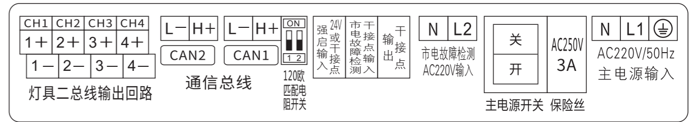
(2)、接线端子说明:
