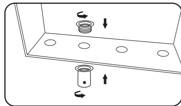
将镀锌管锁母杯梳装进开好的孔上
