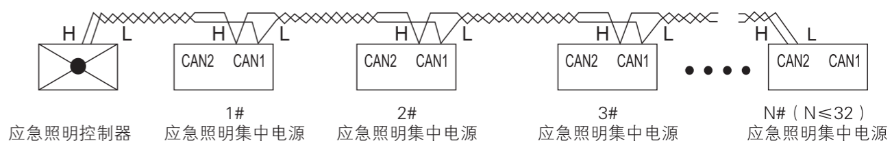
手拉手连接方式示意图（图2）
