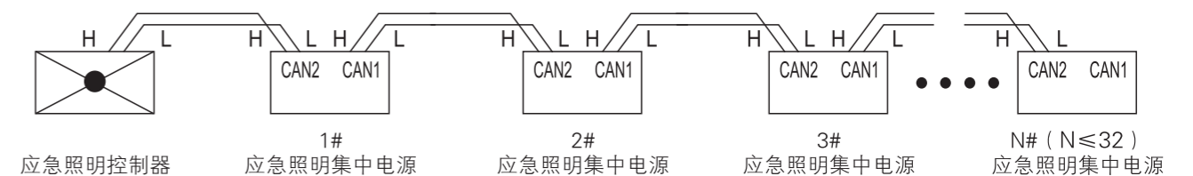
菊花链连接方式示意图（图1）
