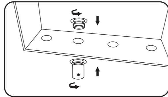
将镀锌管锁母杯梳装进开好的孔上
