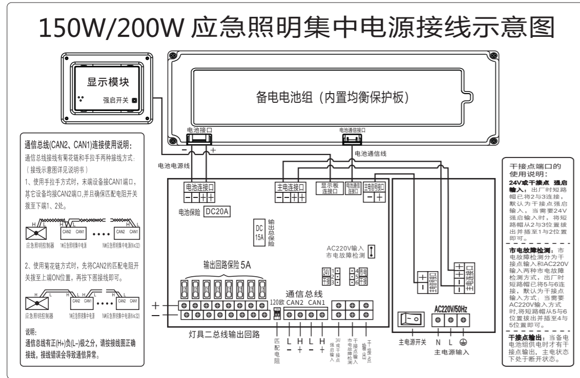
(1)、用户接线示意图 (如图4.1、图4.2)
