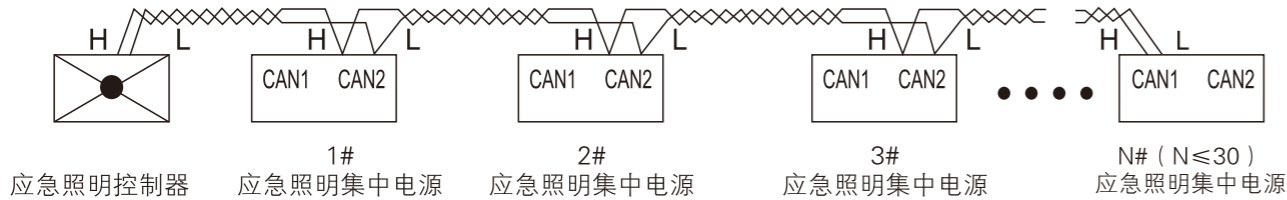
菊花链连接方式示意图（图4.2）
